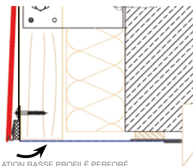
DÉTAIL LINTEAU
